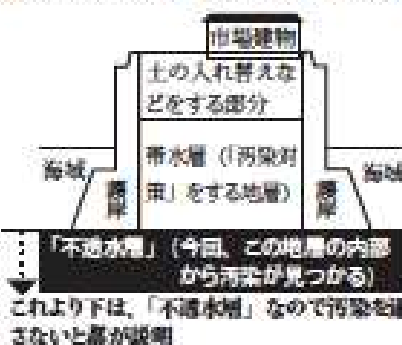
築地の移転予定地－豊洲の土壌(模式図)
